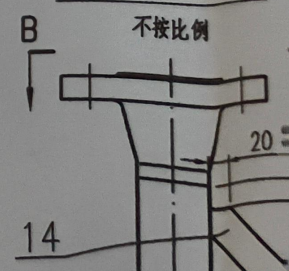
DN \leq 50接管筋板安装详图 不按比例
