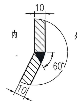
件2与件3焊接详图
