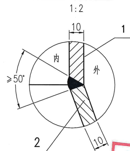
件2与件3焊接详图
