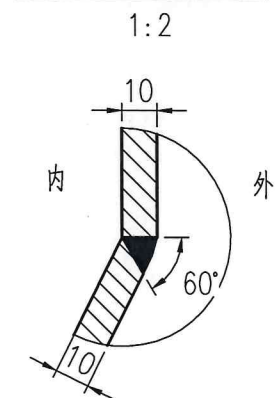
件1与件2焊接详图
